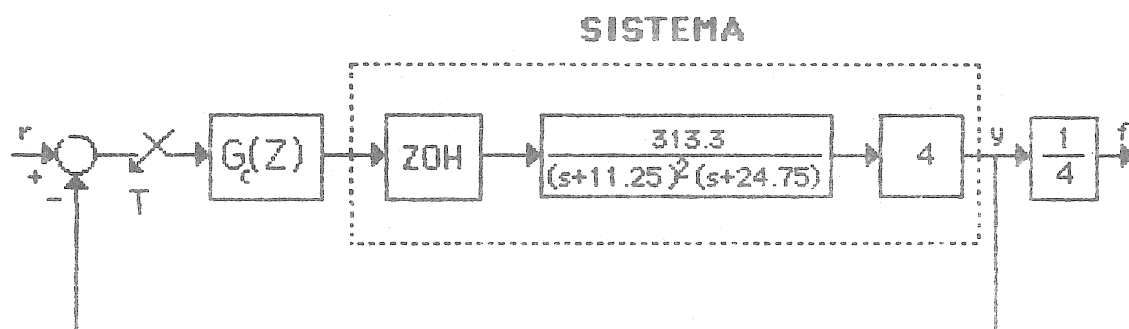
FIGURA 15 Sistema de control realimentado, donde el compensador se encuentran en serie.
