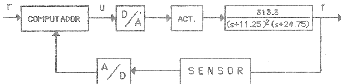
FIGURA 13 Un esquema de implementación digital.
