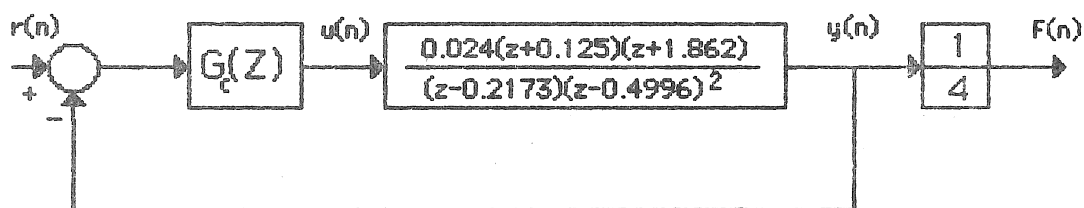
FIGURA 16. Sistema de control discreto.
